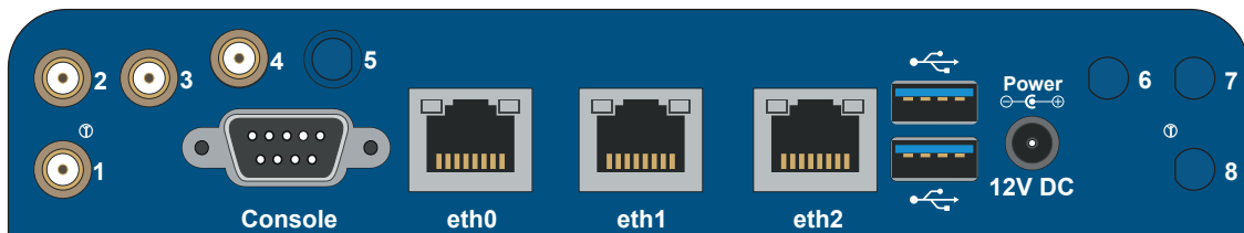
Abb. G3000-5G Rückseite
