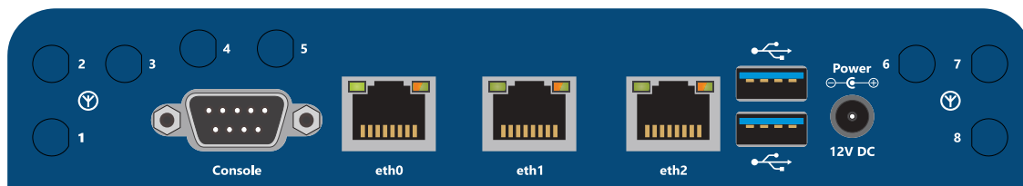
Abb. VA1000-Serie, Rückansicht
